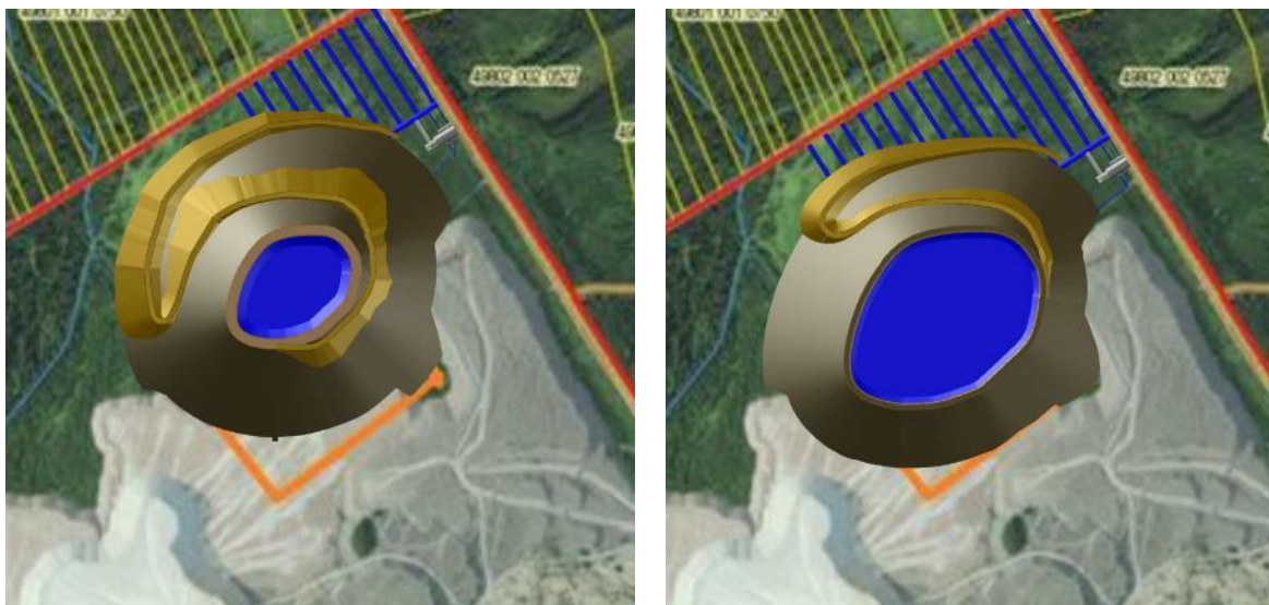
Joonis 3. Illustratiivsed näited maapealse ehitise kõrguse ja veekoguse suhtest (mida kõrgem „mägi“ (vasakpoolsel pildil), seda väiksem maapealne ja maa-alune veereservuaar). Allikas Estonia PHEJ eskiisprojekt
