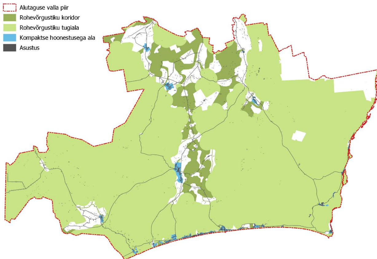
Skeem 11. Alutaguse valla rohevõrgustiku tugialad ja koridorid (Andmed: Maa-amet, 2019).
