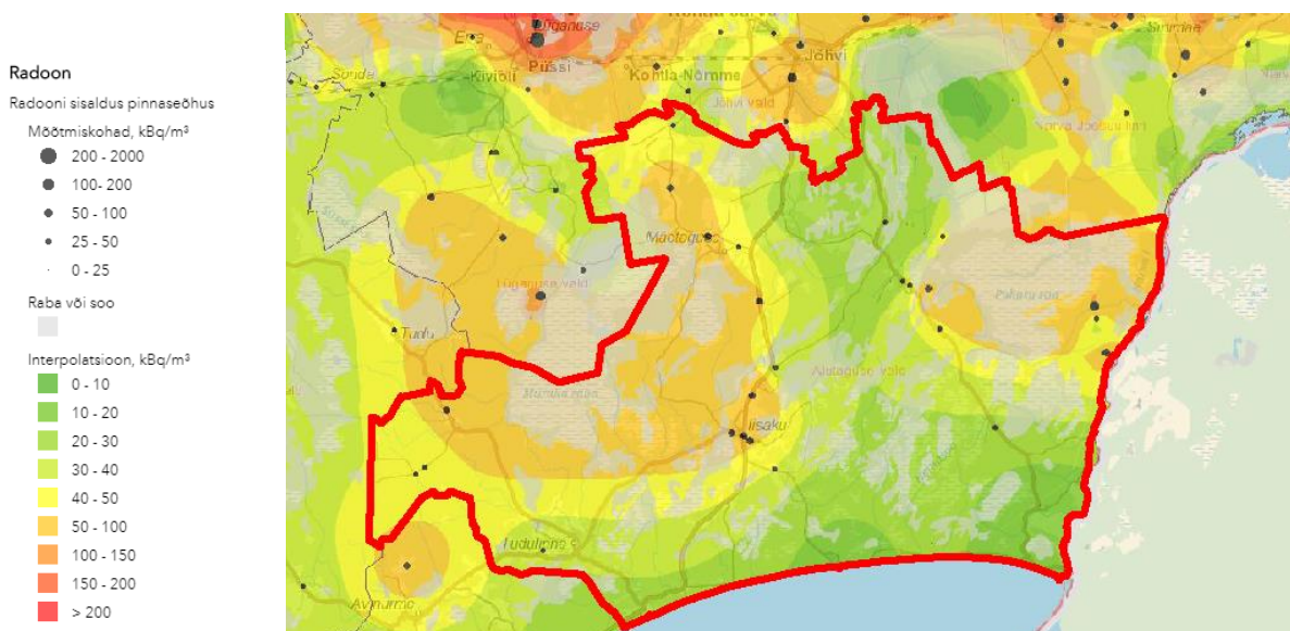
Skeem 7. Väljavõte Eesti radooniriski kaardist (Allikas: Eesti Geoloogiateenistuse kaardirakendus, 04.2018).
