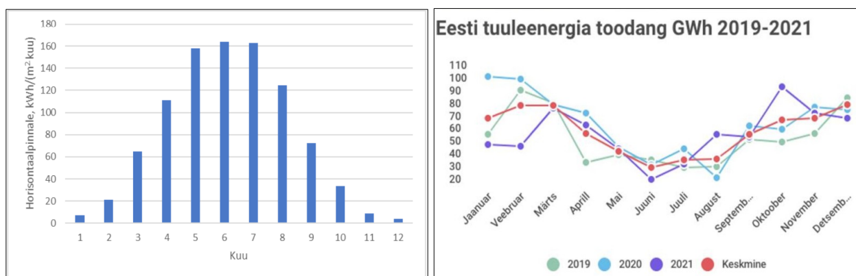
Joonis 10 Päikeseeenergia (Hevac 2020) ja tuuleenergia (Eesti Taastuenergia Assotsiatsioon 2022) efektiivne tootlikus Eestis, kuude lõikes
