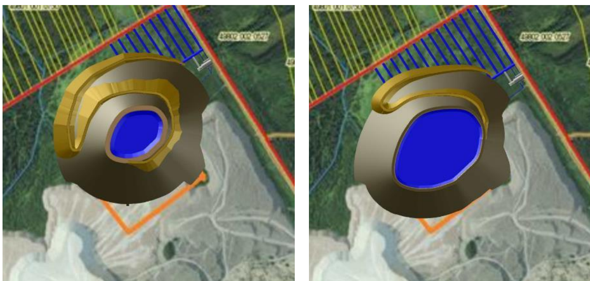
Joonis 3. Illustratiivsed näited maapealse ehitise kõrguse ja veekoguse suhtest (mida kõrgem maapealne alustarind (vasakpoolisel pildil), seda väiksem maapealne ja vastavalt sellele ka maa-alune veereservuaar). Allikas Estonia PHEJ eskiisprojekt
